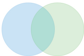
ベン図
